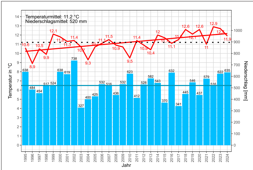
Abb. 7: Jahresmitteltemperaturen und Niederschlagssummen in Gundersheim (1995-2024).
