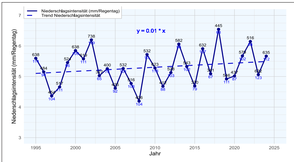
Abb. 21: Niederschlagsintensität pro Jahr (1995-2024) mit Trend.
