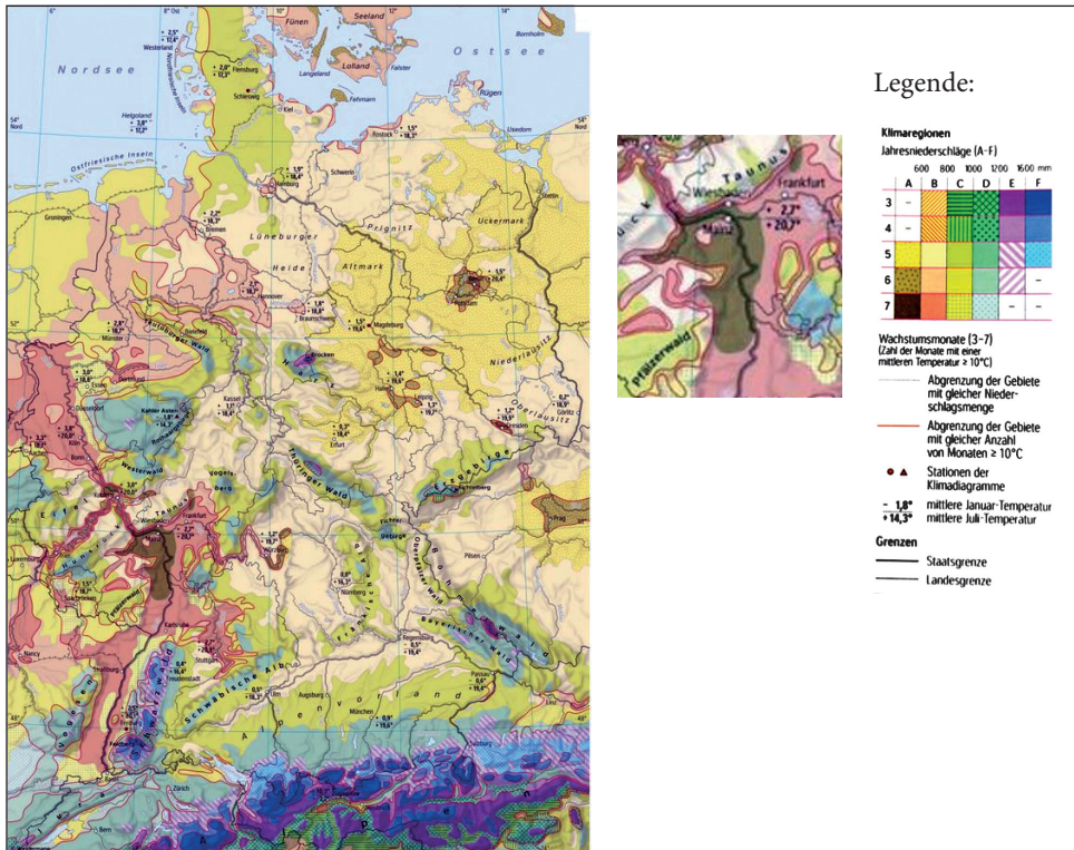
Abb. 2: Klimaregionen Deutschlands mit einem Detailausschnitt der Region um Gundersheim. Der Nördliche Oberrheingraben gehört zur Kategorie A7 mit durchschnittlichen Jahresniederschlägen unter 600 mm (A) und sieben Monaten mit Durchschnittstemperaturen über 10 °C (aus: Diercke Weltatlas, 2023).
