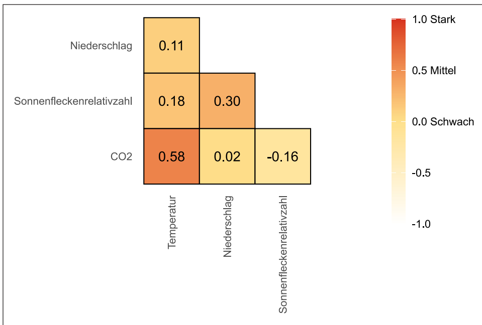
Abb. 25: Korrelationskoeffizienten der Variablen Temperatur, Niederschlag, Sonnenfleckenrelativzahl und CO 2 . Quellen: Meteo.Plus/ Umweltbundesamt.
