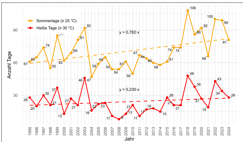
Abb. 18: Anzahl der heißen Tage und Sommertage pro Jahr (1995-2024) mit Trendlinie.
