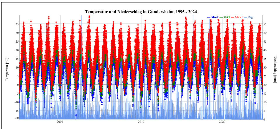
Abb. 8: Temperatur und Niederschlag in Gundersheim, Tageswerte vom 1.1.1995 bis 31.12.2024.
