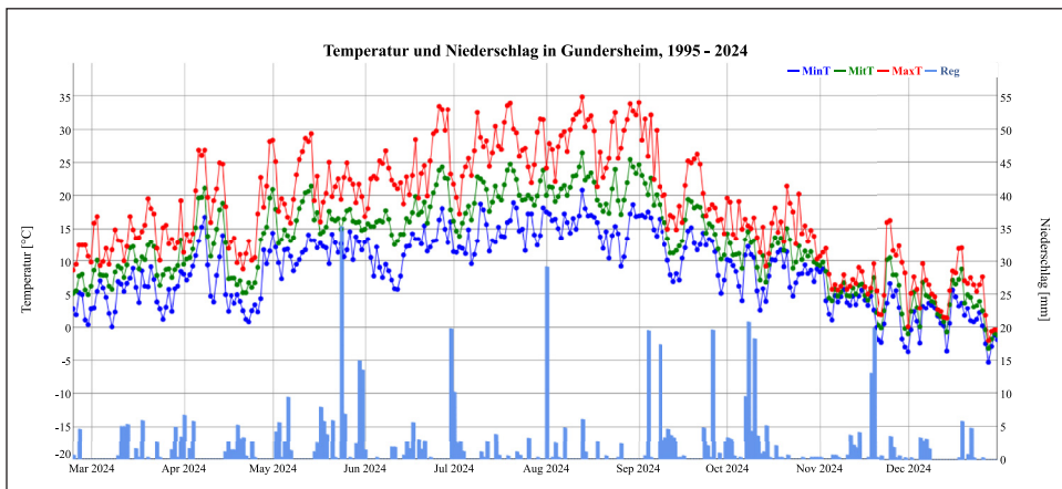
Abb. 9: Temperatur und Niederschlag in Gundersheim von März bis Dezember 2024.
