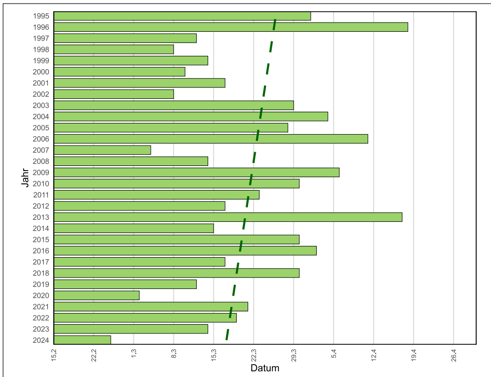
Abb. 28: Darstellung des Termins des Erreichens der Wärmesumme von 200 °C mit eingezeichneter Trendlinie, 1925-2024.
