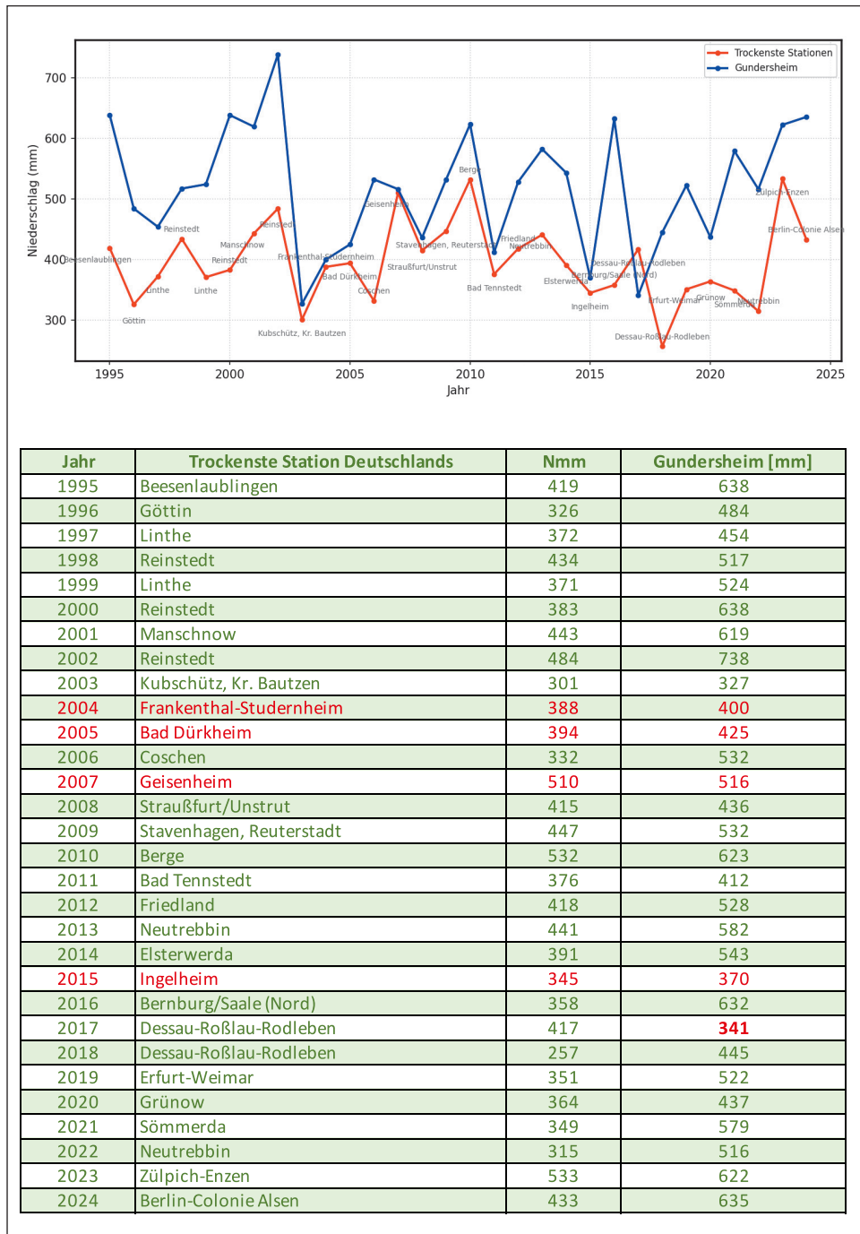
Abb. 16: Liste der Jahresniederschlagssummen der trockensten Stationen Deutschlands 1995-2024 im Vergleich zu Gundersheim. Rechts: Vergleich des Niederschlags: Trockenste Stationen vs. Gundersheim.
