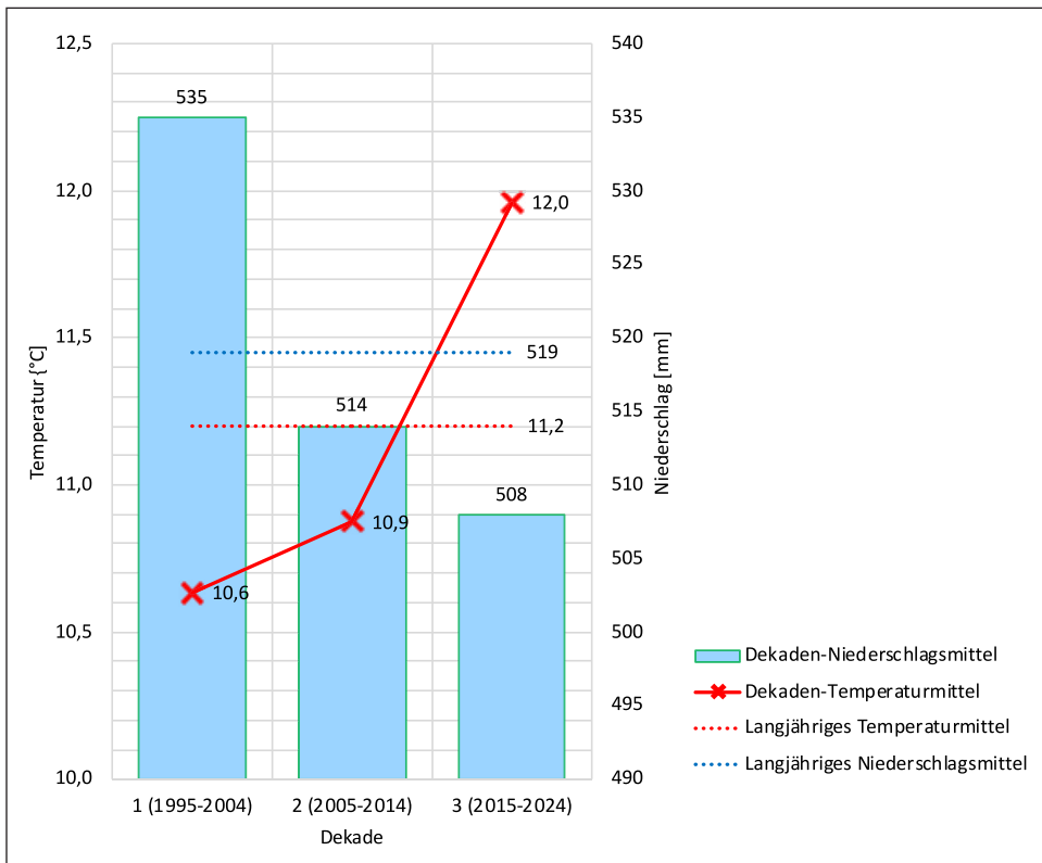
Abb. 10: Vergleich der Dekaden zu den langjährigen Mittelwerten von Temperatur und Niederschlag in Gundersheim für den Beobachtungszeitraum 1995-2024.
