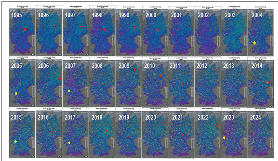
Abb. 15: Jahresniederschlagssummen in Deutschland, 1995-2024. Roter Punkt: Station des niedrigsten Jahresniederschlags (Ostdeutschland). Gelber Punkt: Station des geringsten Jahresniederschlags (Oberheingraben). Quelle: Deutscher Wetterdienst.
