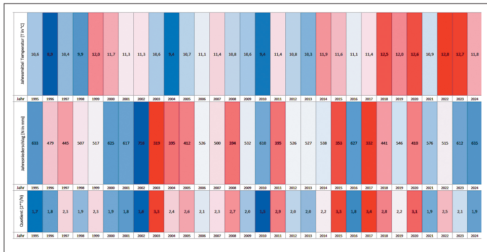
Abb. 5: Zeitreihenvergleich der Jahresmitteltemperaturen und -niederschläge für Gundersheim.
