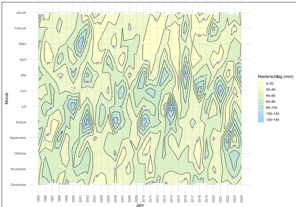
Abb. 6: Monatliche Niederschlagssummen für den Zeitraum von 1995-2024 in Gundersheim.
