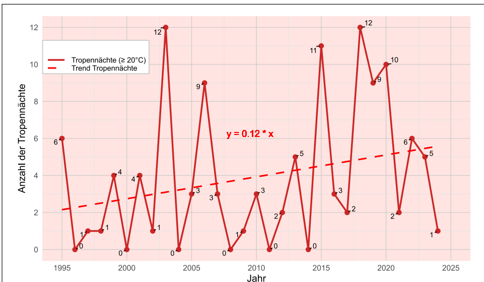
Abb. 20: Anzahl der Tropennächte pro Jahr (1995-2024) mit Trend.
