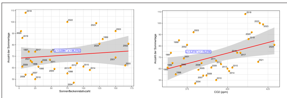
Abb. 24: Korrelation zwischen Sonnenflecken und Sommertagen mit Trend und 95%-Konfidenzbereich (1995-2024), r=0,12 , p=0,52 (links). Korrelation zwischen CO 2 und Sommertagen mit Trend und 95%-Konfidenzbereich (1995-2024), r=0,45 , p=0,0124 (rechts).
