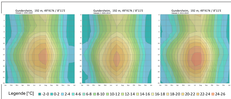
Abb. 13: Thermoisoplethendiagramme der drei Dekaden. Links: Dekade 1 (1995-2004), Mitte: Dekade 2 (2005-2014), Rechts: Dekade 3 (2015-2024).
