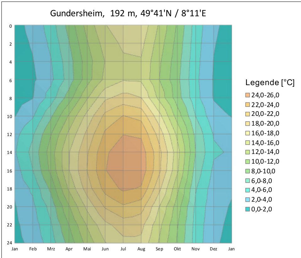
Abb. 12: Thermoisoplethendiagramm von Gundersheim, 193 m ü. NHN, 49°41'N / 8°11'E.
