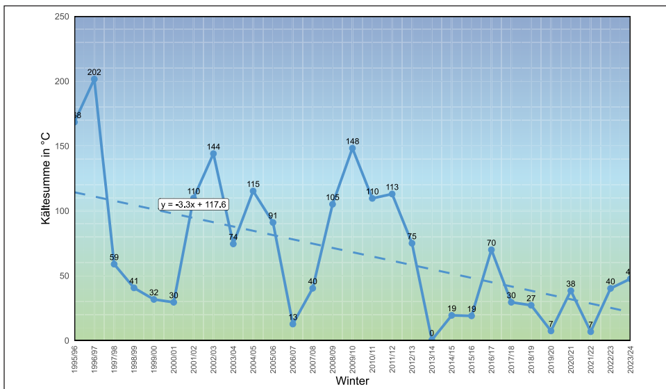
Abb. 26: Summe der negativen Tagesmittel (Kältesumme) pro Winter (Dezember-Februar), 1995-2024.
