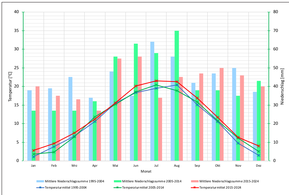
Abb. 11: Vergleich der Temperaturmittel und Niederschlagssummen in Gundersheim nach Dekaden.
