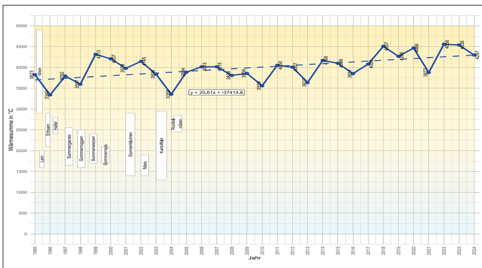
Abb. 27: Summe der Tagesmittel-Temperaturwerte (Wärmesumme) in der Vegetationsperiode ( \geq 5\text{ }^{\circ}\text{C} ), 1995-2024.
