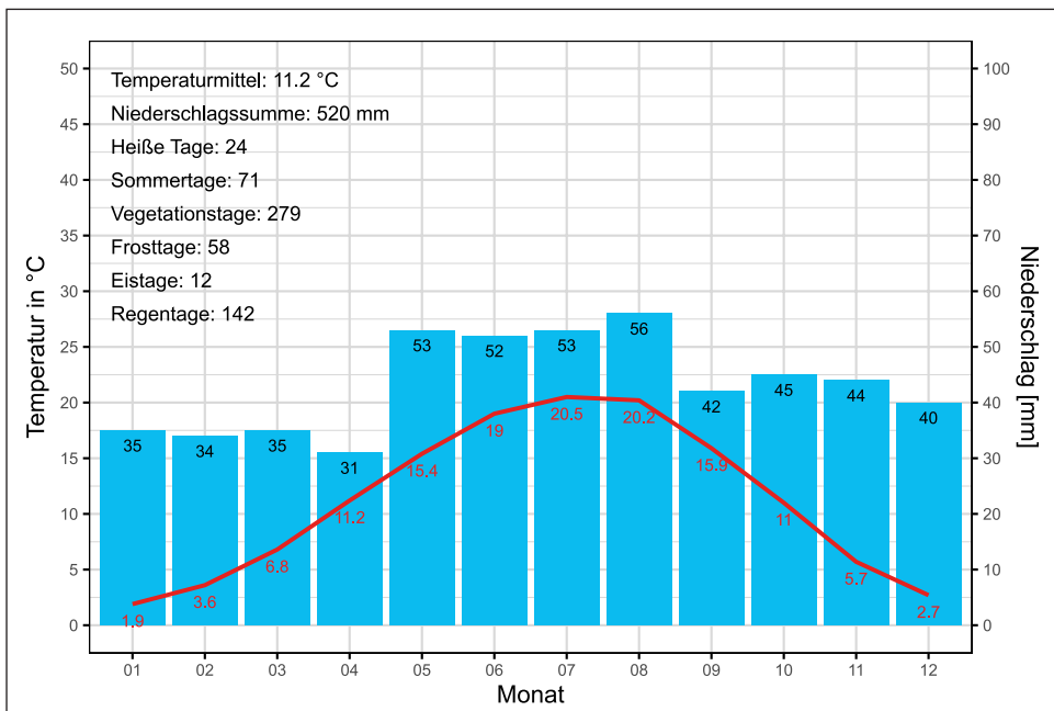
Abb. 4: Klimadiagramm von Gundersheim, 193 m ü. NHN (1995-2024) nach WALTER & LIETH.
