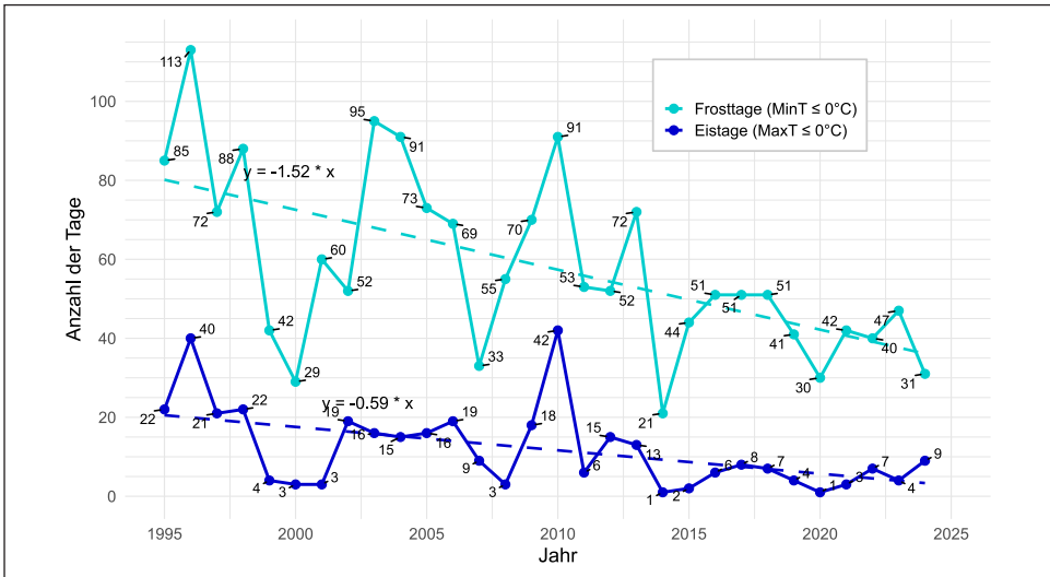
Abb. 19: Anzahl der Frost- und Eistage pro Jahr (1995-2024) mit Trend.
