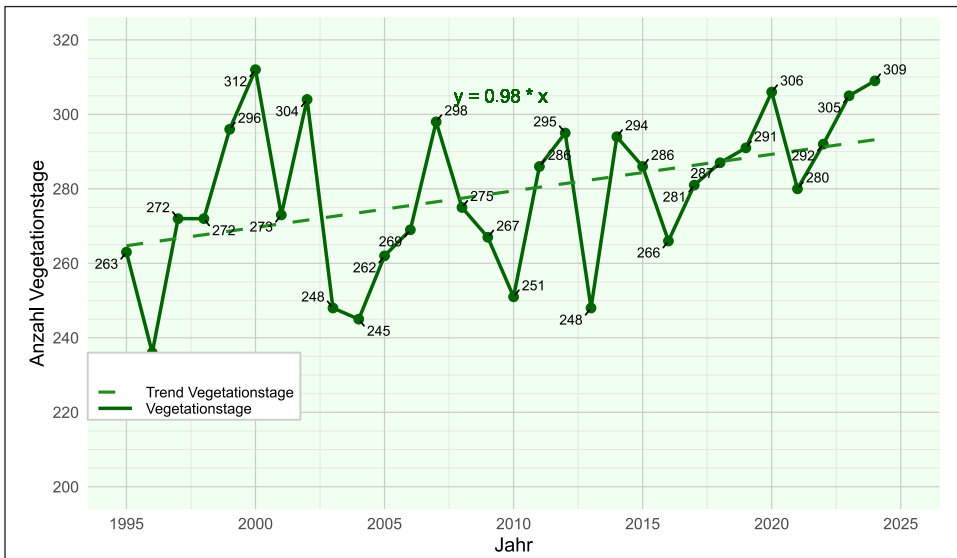
Abb. 22: Vegetationstage pro Jahr (1995-2024) mit Trend
